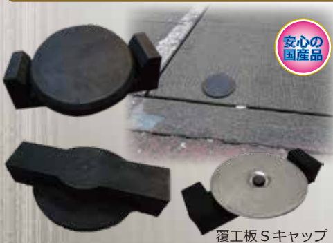
覆工板 S キャップ
